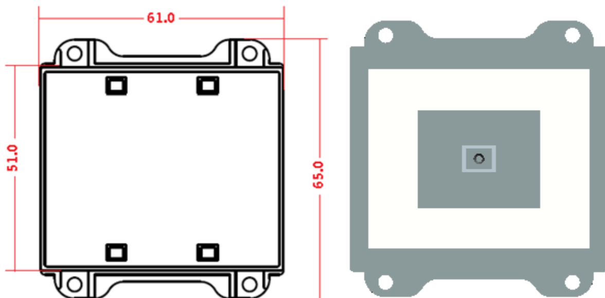
NT351J 前视图（单位：mm）
