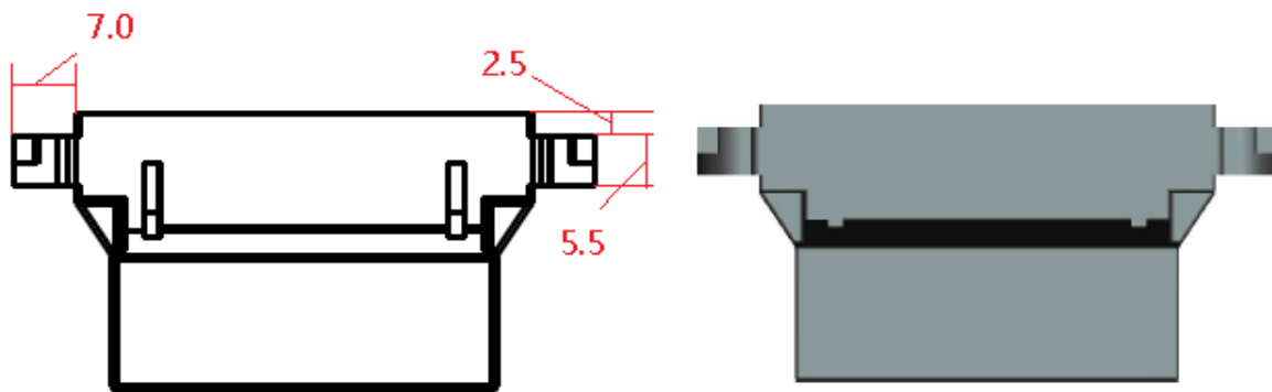
NT351J 俯视图 (单位 : mm)
