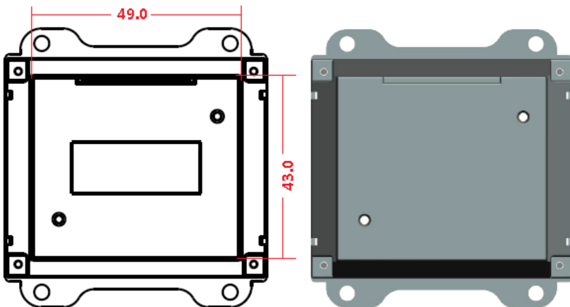
NT351J 俯视图 (单位 : mm)
