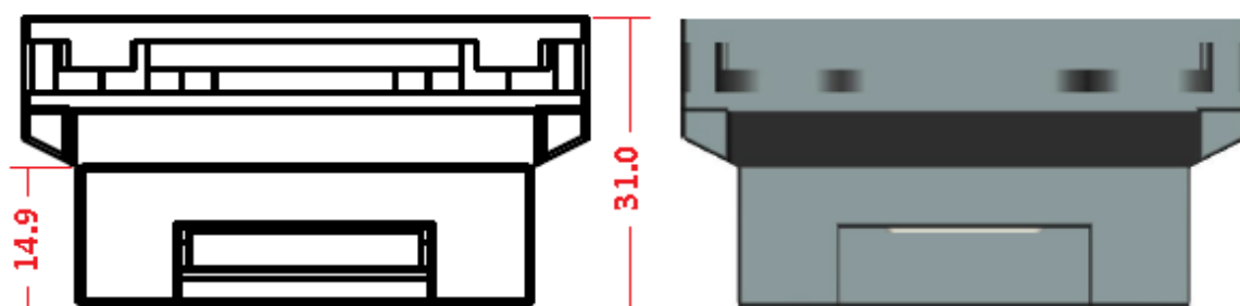
NT351J 侧视图（单位：mm）
